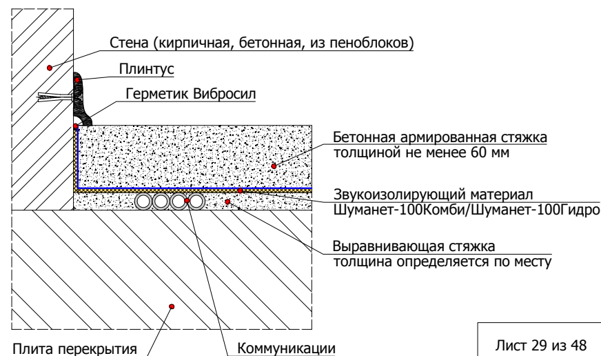
6.2.4 Схема примыкания конструкции плавающего пола с применением звукоизолирующего материала Шуманет-100Комби/Шуманет-100Гидро к стене и коммуникациями под стяжкой
