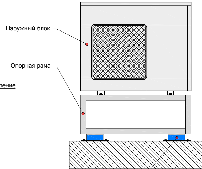
7.2.3 Схема закрепления наружного блока системы кондиционирования с применением виброизоляционных креплений Виброфлекс-EP/25
