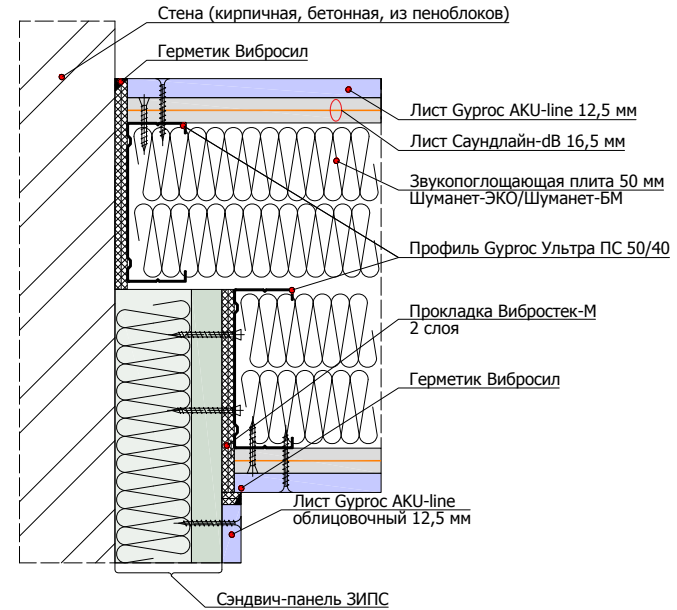
1.6.4 Угловое примыкание перегородки на двойном 2x100 мм (независимом) каркасе к панелям ЗИПС на стене
