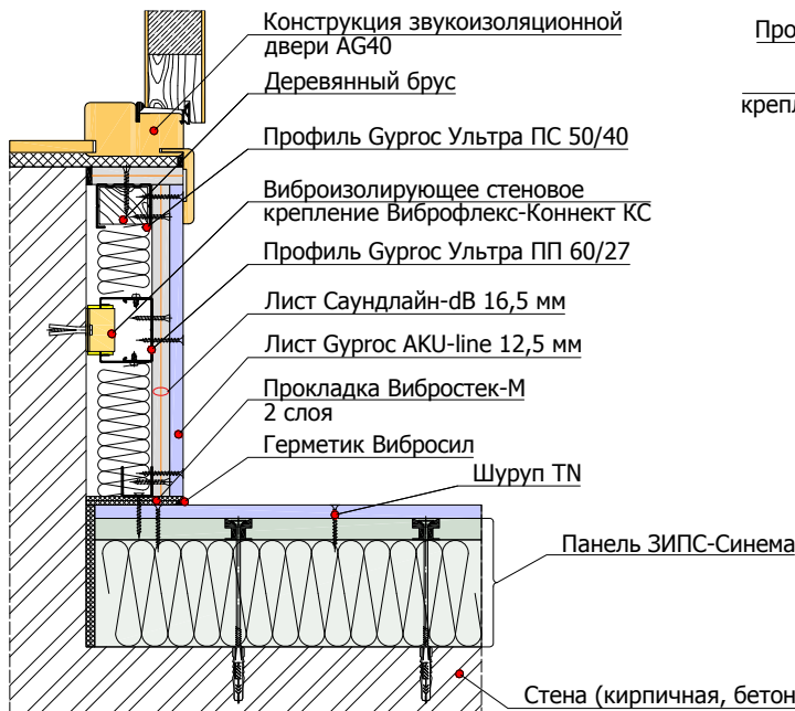
4.5.3 Угловое примыкание облицовки стены на каркасе ПП 60/27 и виброизолирующих стеновых креплениях Виброфлекс-КС к панелям ЗИПС на стене и дверному проему
