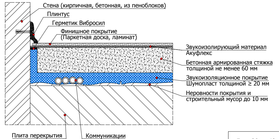
6.1.4 Схема применения материала Акуфлекс под финишным покрытием в сочетании с конструкцией плавающего пола с применением звукоизолирующего материала Шумопласт
