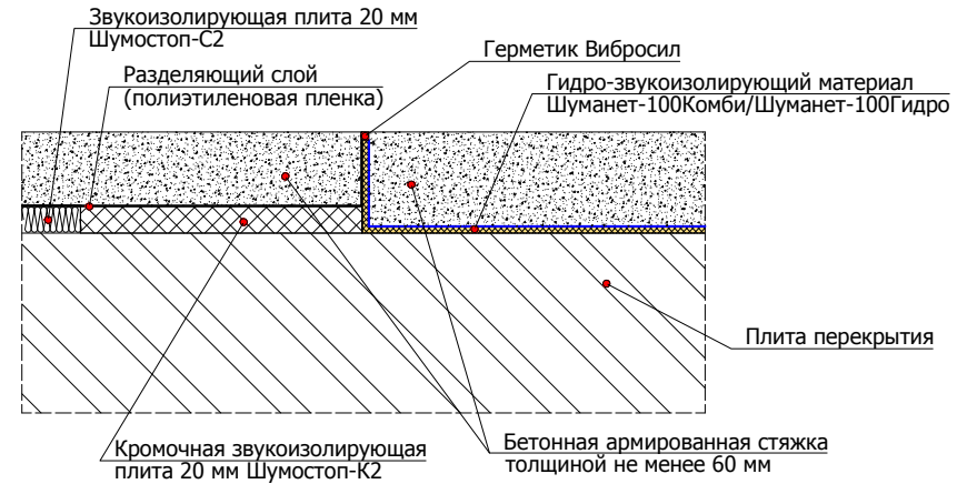
6.2.8 Схема примыкания конструкции плавающего пола с применением звукоизолирующего материала Шуманет-100Комби/Шуманет-100Гидро к стене
