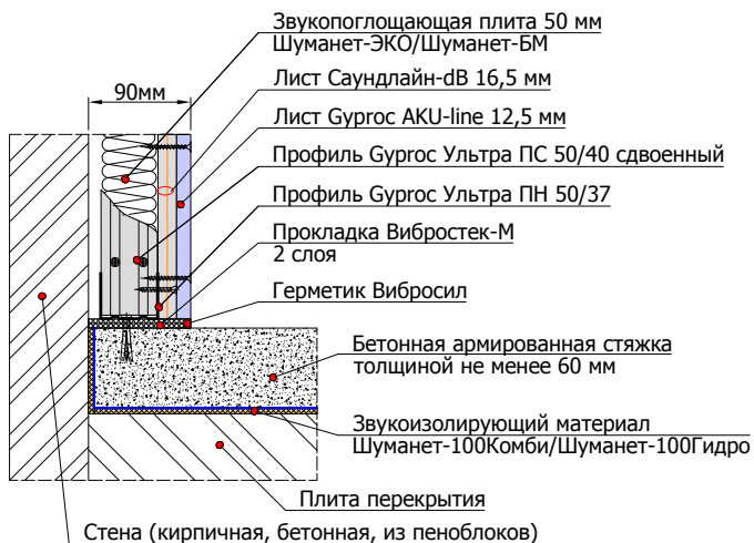
4.2.1 Примыкание облицовки стены на независимом сдвоенном каркасе 50 мм к конструкции "плавающего" пола
