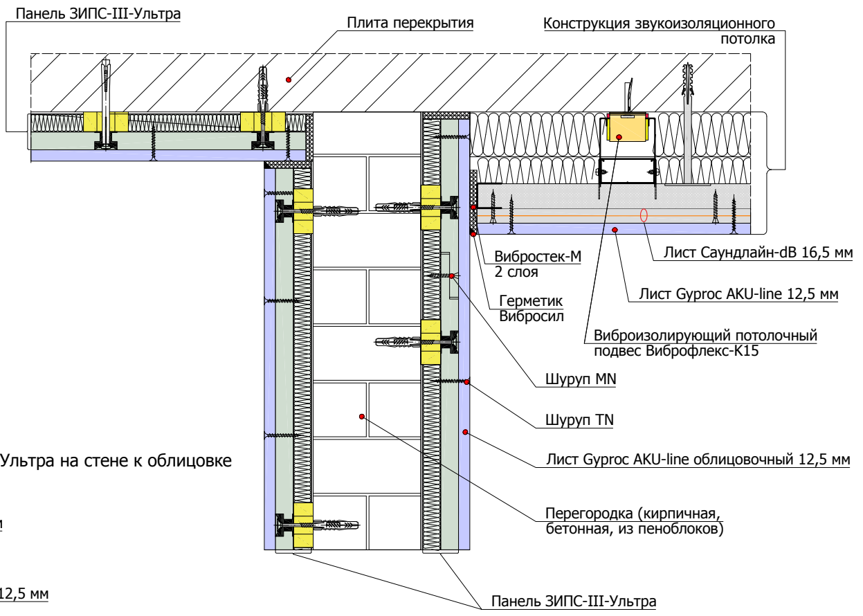
2.5.1 Примыкание панелей ЗИПС-III-Ультра к перекрытию пола/потолка
