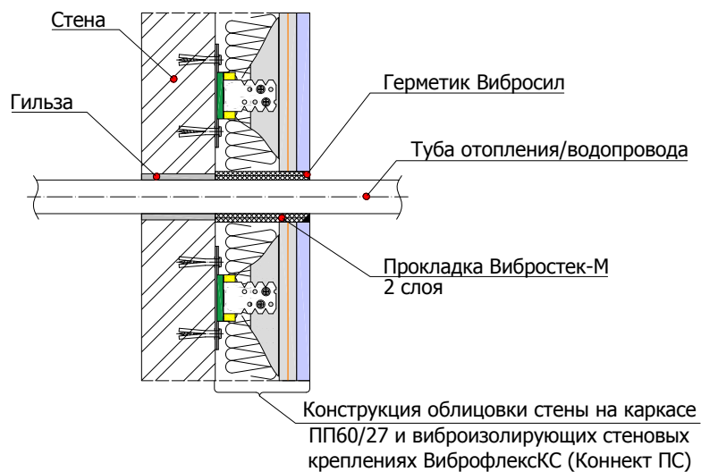
8.5.3 Схема пропуска труб отопления/водопровода через конструкцию облицовки стены на каркасе ПП 60/27 и виброизолирующих стеновых креплениях Виброфлекс-КС (Коннект ПС)
