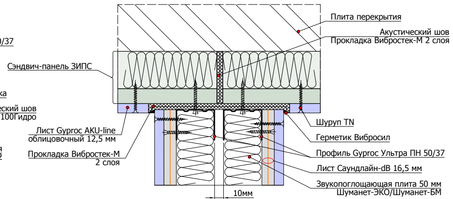
1.4.2 Примыкание перегородки на двойном 2x50 мм (независимом сдвоенном) каркасе к панелям ЗИПС
