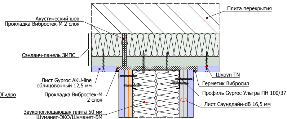
1.2.6 Примыкание перегородки на одинарном каркасе 100 мм к панелям ЗИПС на потолочном перекрытии
