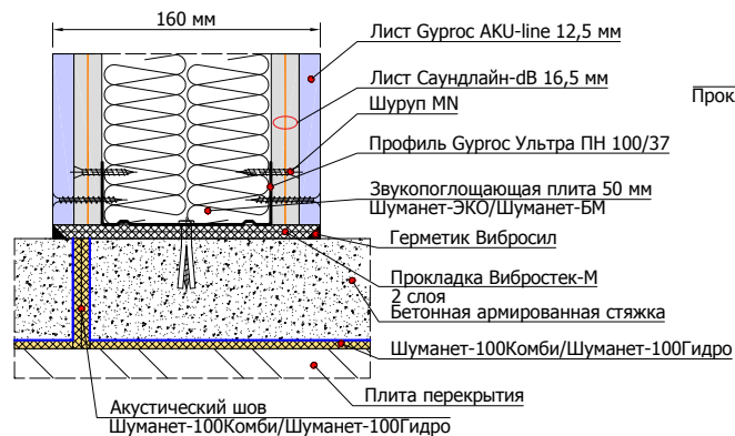
1.2.5 Примыкание перегородки на одинарном каркасе 100 мм к конструкции "плавающего" пола
