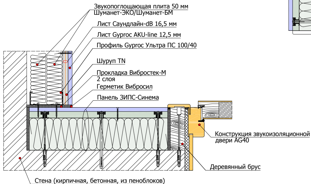
2.4.3 Угловое примыкание панелей ЗИПС-Синема на стене к облицовке на каркасе 100 мм и дверному проему
