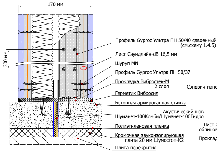
1.4.1 Примыкание перегородки на двойном 2x50 мм (независимом сдвоенном) каркасе к конструкции "плавающего" пола
