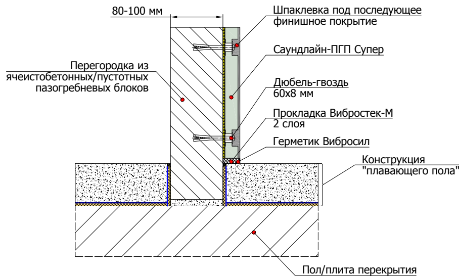
3.3 Примыкание конструкции "плавающего пола" к панелям Саундлайн-ПГП Супер, смонтированным на перегородку из ячеистобетонных/пустотных пазогребневых блоков
