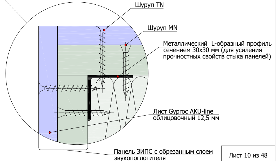
2.1.5 Узлы крепления панелей ЗИПС при монтаже внешнего угла
