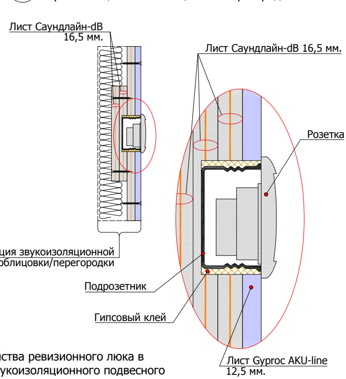
8.2.1 Схема устройства встроенных розеток в конструкциях звукоизоляционных облицовок и перегородок
