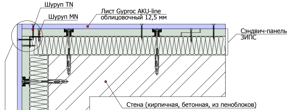
2.1.3 Монтаж панельной системы ЗИПС на внешний угол (горизонтальный разрез)
