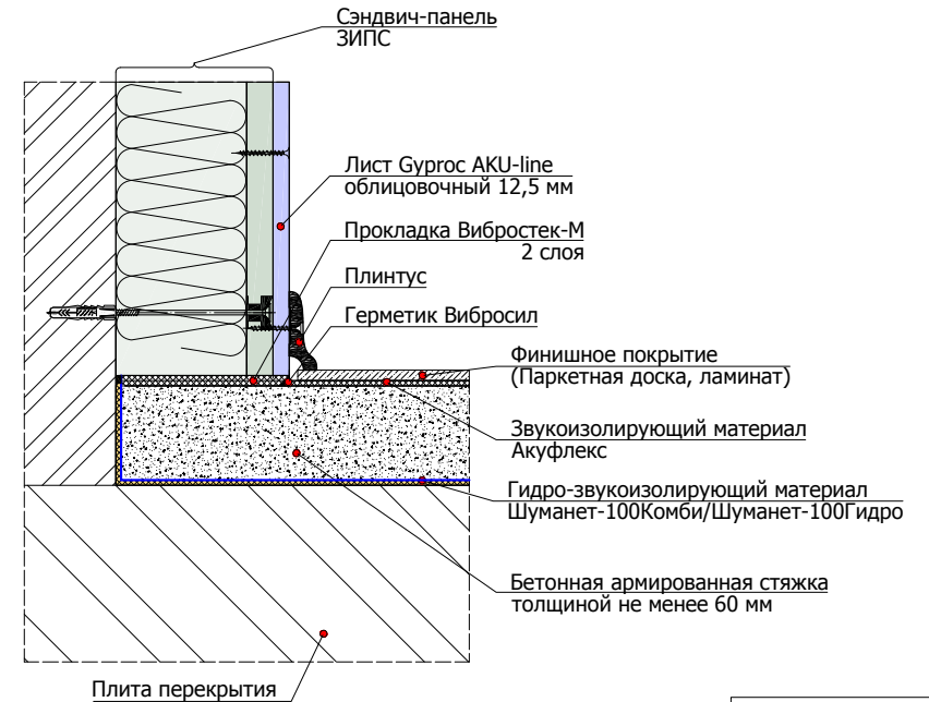
6.2.8 Схема примыкания конструкции плавающего пола с применением звукоизолирующего материала Шуманет-100Комби/Шуманет-100Гидро к стене
