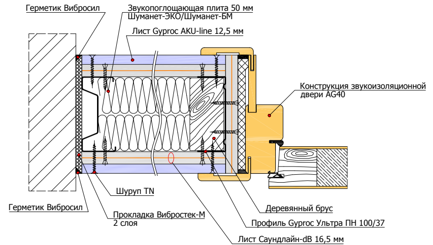
1.4.2 Примыкание перегородки на двойном 2x50 мм (независимом сдвоенном) каркасе к панелям ЗИПС
