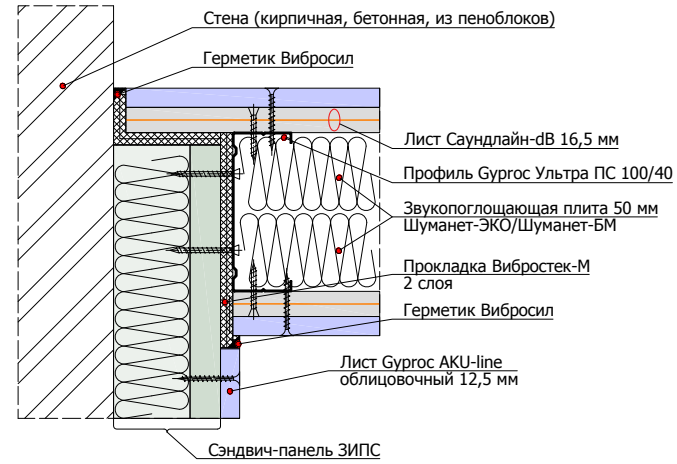
1.6.4 Угловое примыкание перегородки на двойном 2x100 мм (независимом) каркасе к панелям ЗИПС на стене
