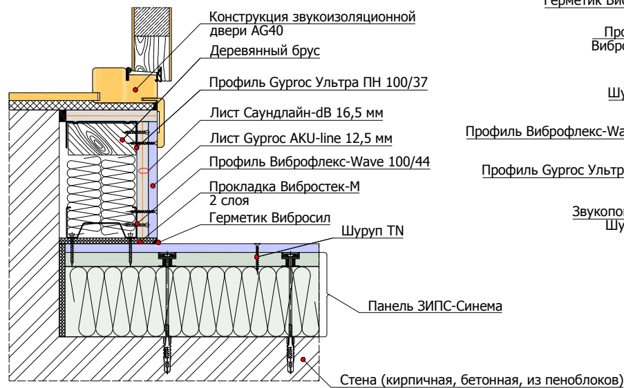
4.3.3 Угловое примыкание облицовки стены на независимом каркасе из профилей Виброфлекс-Wave 100 мм к панелям ЗИПС на стене и дверному проему
