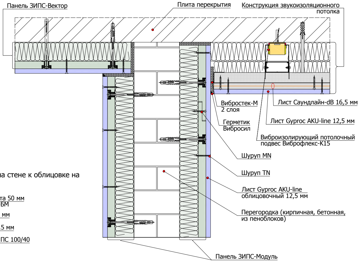
2.3.2 Примыкание панелей ЗИПС-Модуль к панелям ЗИПС-Модуль на потолочном перекрытии и подвесному звукоизолирующему потолку
