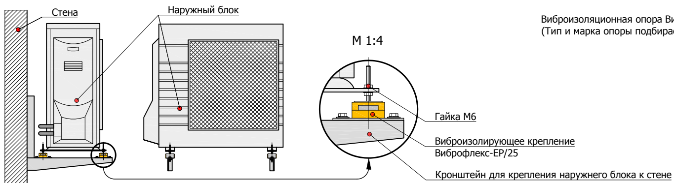
7.2.3 Схема закрепления наружного блока системы кондиционирования с применением виброизоляционных креплений Виброфлекс-EP/25
