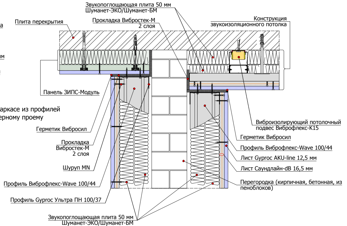
4.3.2 Примыкание облицовки стены на независимом каркасе из профилей Виброфлекс-Wave 100 мм к панелям ЗИПС на потолочном перекрытии и подвесному звукоизолирующему потолку
