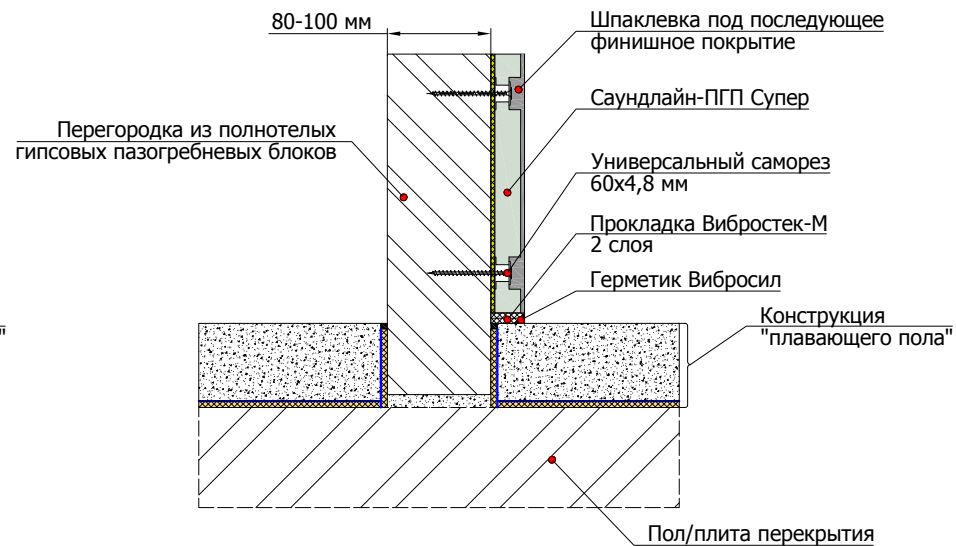
3.4 Примыкание конструкции "плавающего пола" к панелям Саундлайн-ПГП Супер, смонтированным на перегородку из полнотелых гипсовых пазогребневых блоков
