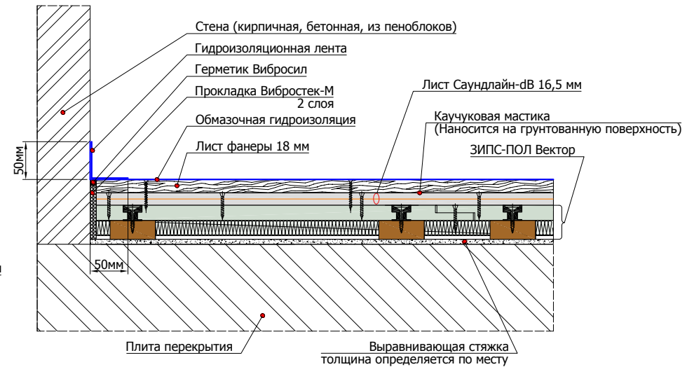
6.8.4 Схема устройства гидроизоляции в конструкции пола с применением панелей ЗИПС-ПОЛ
