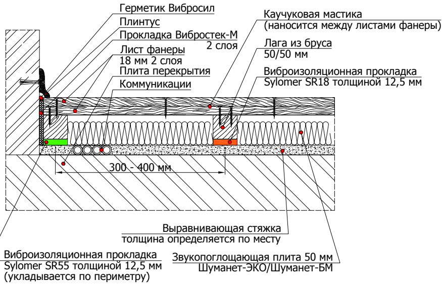
6.7.3 Схема примыкания конструкции пола по деревянным лагам с применением виброизоляционного материала Sylomer к стене и трубе отопления/водопровода (монтаж на ровное перекрытие)
