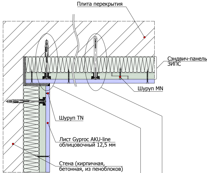
2.1.2 Монтаж панельной системы ЗИПС (вертикальный разрез)
