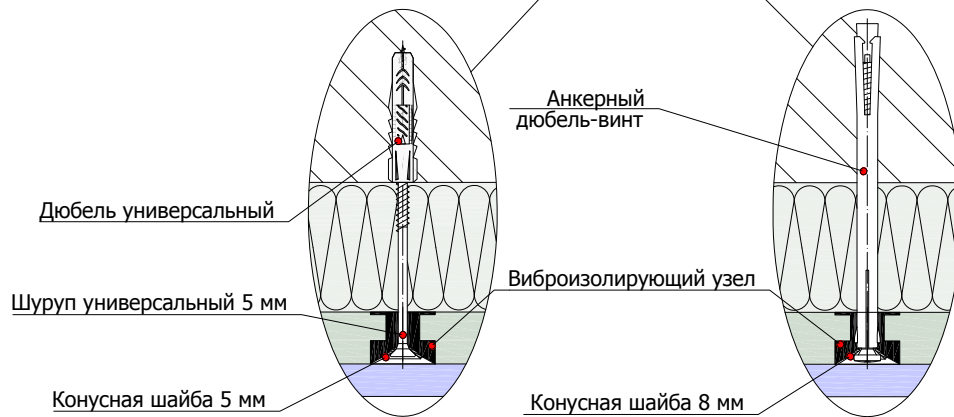
2.1.4 Узлы крепления панелей ЗИПС
