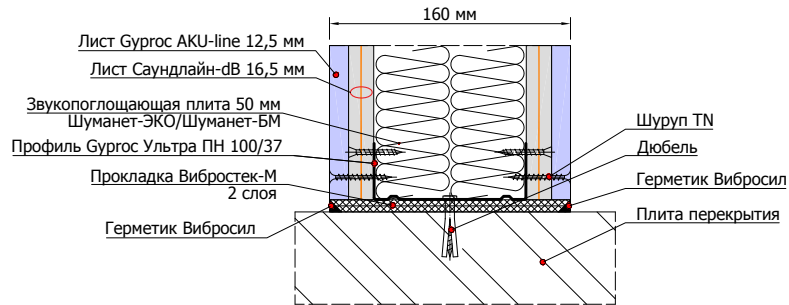
1.3.5 Примыкание перегородки на одинарном каркасе из профилей Виброфлекс-Wave 100 мм к перекрытию пола/потолка
