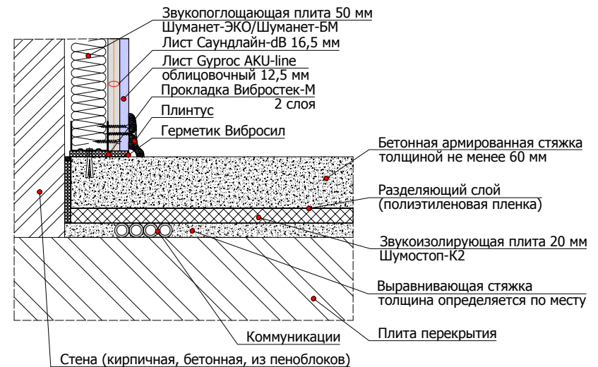
6.4.4 Схема примыкания конструкции плавающего пола с применением звукоизолирующих плит Шумостоп-K2 в один слой к стене и коммуникациями под стяжкой
