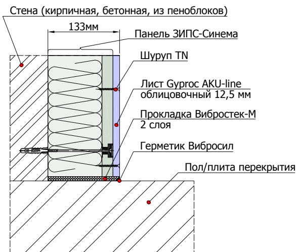
2.4.1 Примыкание панелей ЗИПС-Синема к перекрытию пола/потолка
