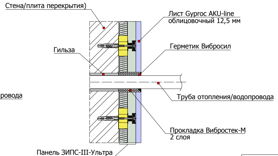
8.4.4 Схема пропуска труб отопления/водопровода через конструкцию панельной системы ЗИПС-III-Ультра
