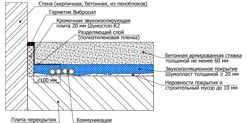
6.5.4 Схема устройства конструкции плавающего пола с коммуникациями под стяжкой с применением звукоизолирующего покрытия Шумопласт
