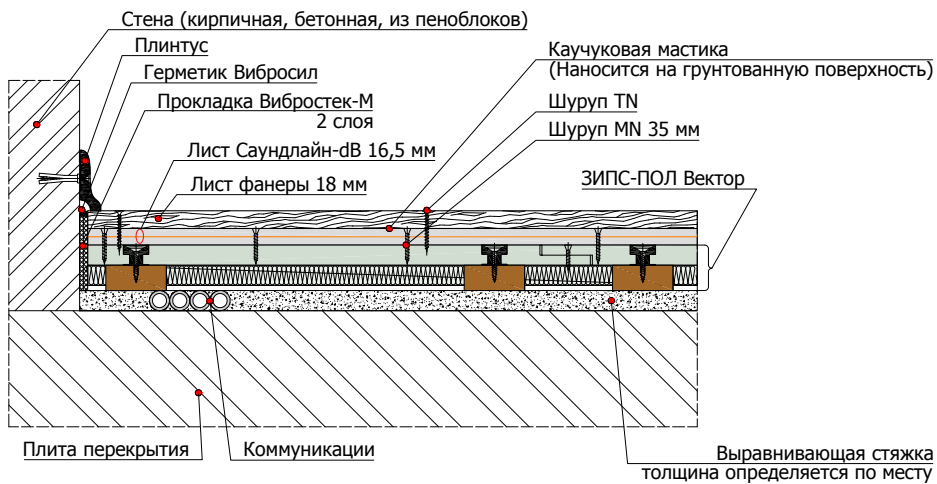
6.6.1 Схема устройства конструкции ЗИПС-ПОЛ Вектор
