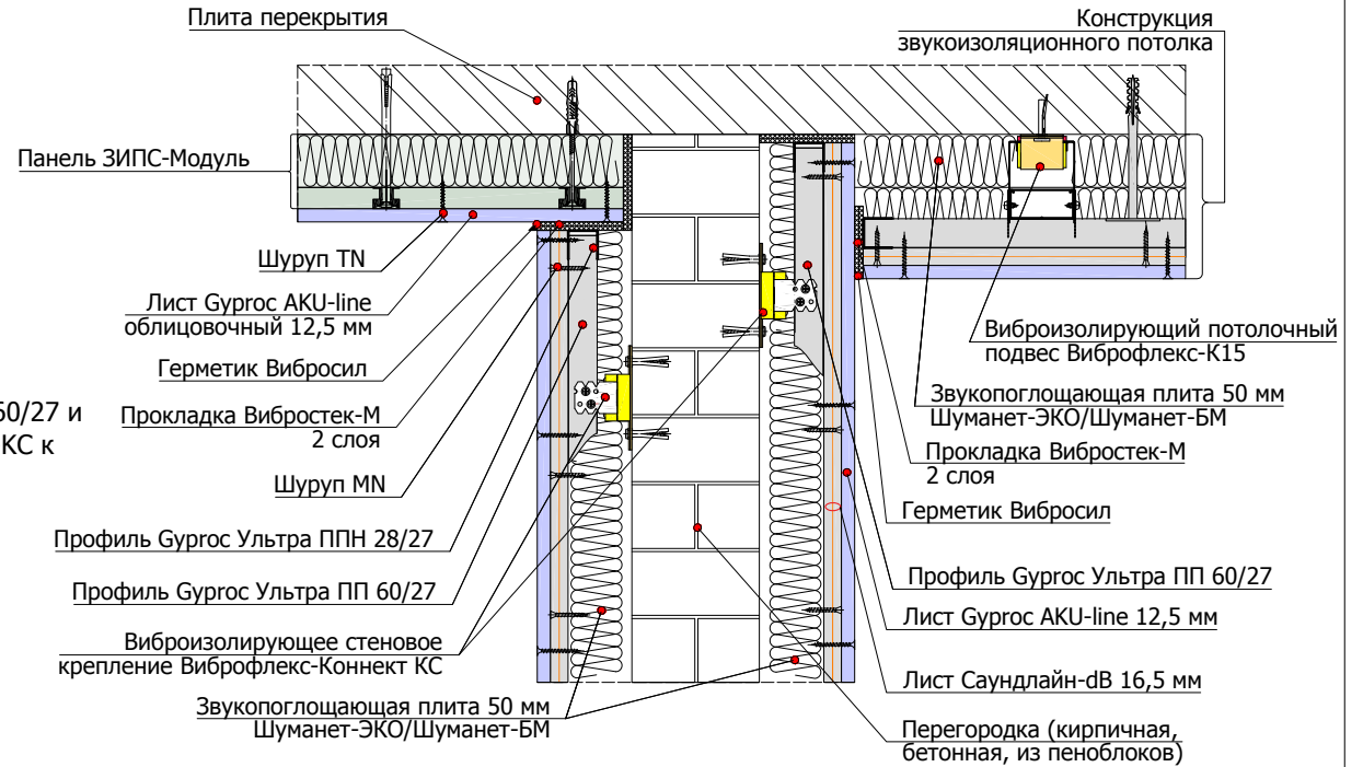
4.5.2 Примыкание облицовки стены на каркасе ПП 60/27 и виброизолирующих стеновых креплениях Виброфлекс-КС к панелям ЗИПС на потолочном перекрытии и к подвесному звукоизолирующему потолку
