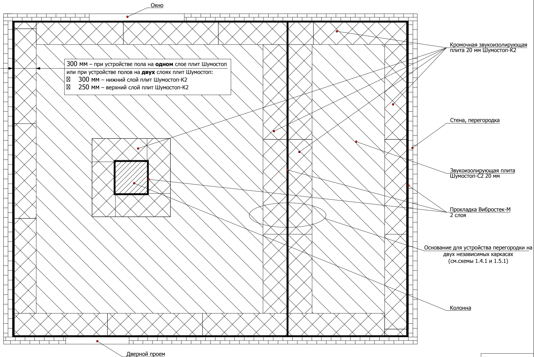
6.3.9 Схема устройства конструкции звукоизоляционного пола плавающего типа с применением звукоизолирующих плит Шумостоп (вид в плане)
