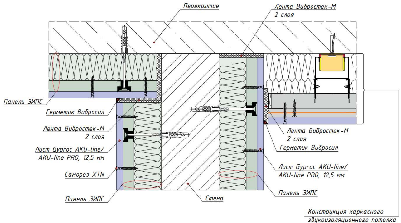
Рисунок 15. Угловое примыкание панельной системы ЗИПС к панельной системе ЗИПС/ каркасному звукоизоляционному потолку на перекрытии.
